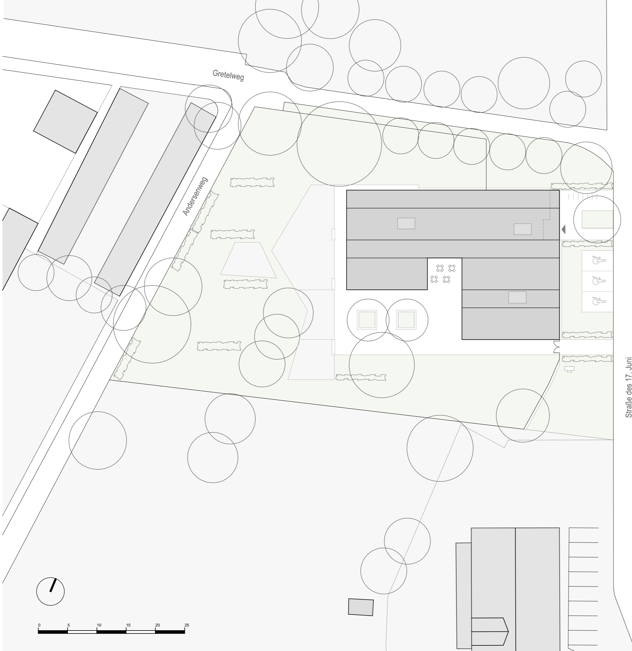
Betriebskindergarten "Gipfelstürmer" Weimar, Lageplan M 1:400
